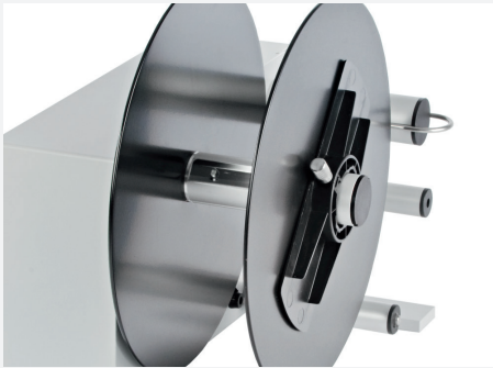
Etikettenaufwickelvorrichtung Label rewinder
